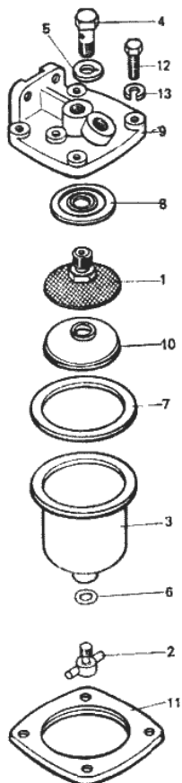
Рис. 24. Фильтр топливный грубой очистки А23.20.000-01
